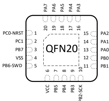
图 3-2 QFN20 Pinout1 PY32L020F15U
