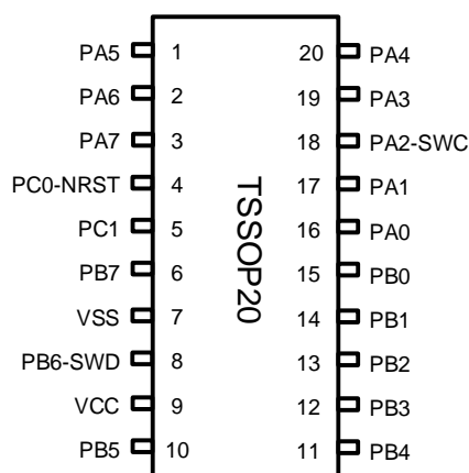
图 3-1 TSSOP20 Pinout1 PY32L020F15P
