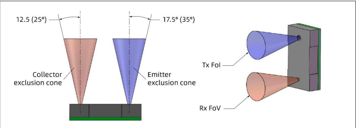
图 12：XL5300 FoI/FoV
