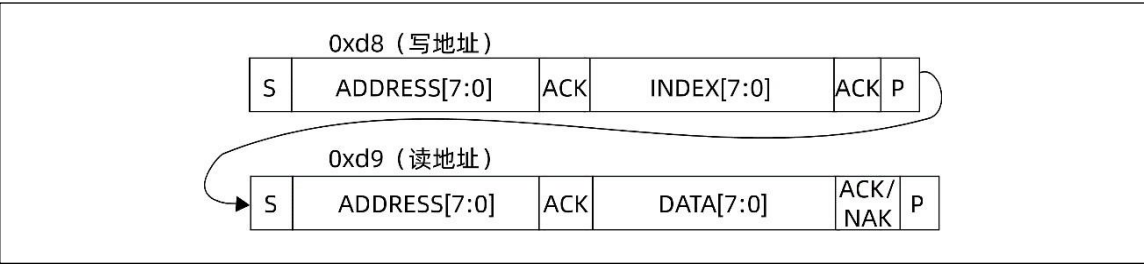
图 7 : XL5300 读数据格式
