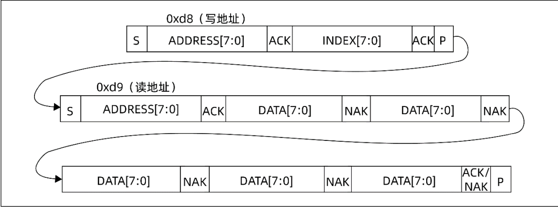
图 9 : XL5300 连续读数据格式
