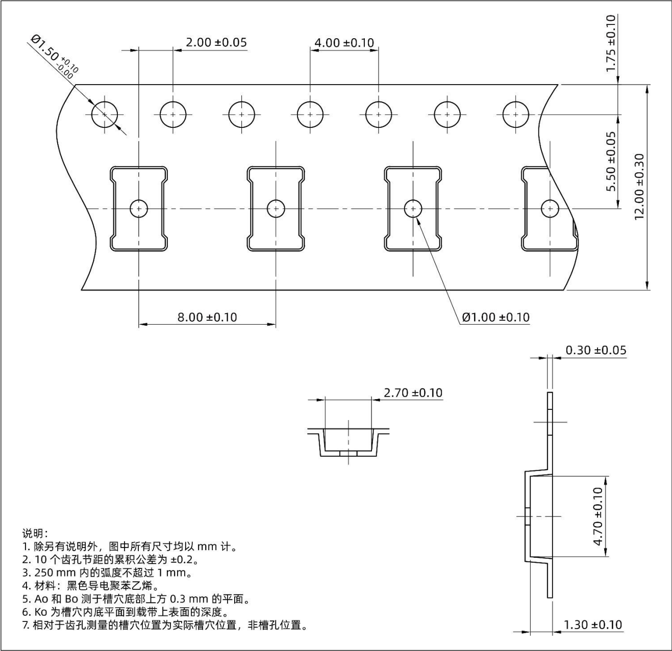
图 16：卷带尺寸图
