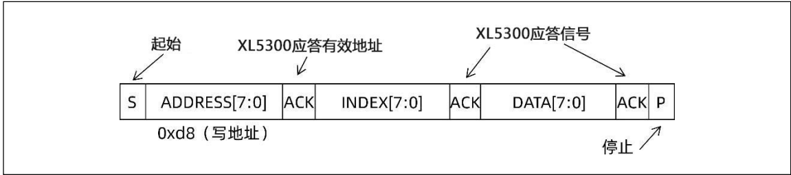
图 6 : XL5300 写数据格式
