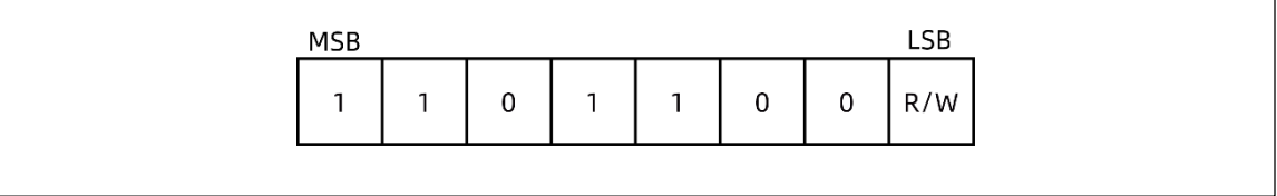
图 5：XL5300 I 2 C 器件地址 0xd8
