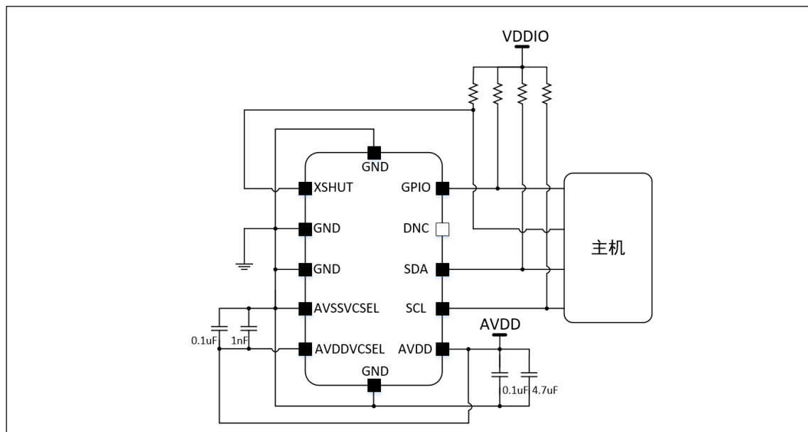
图 13 : XL5300 电路框图
