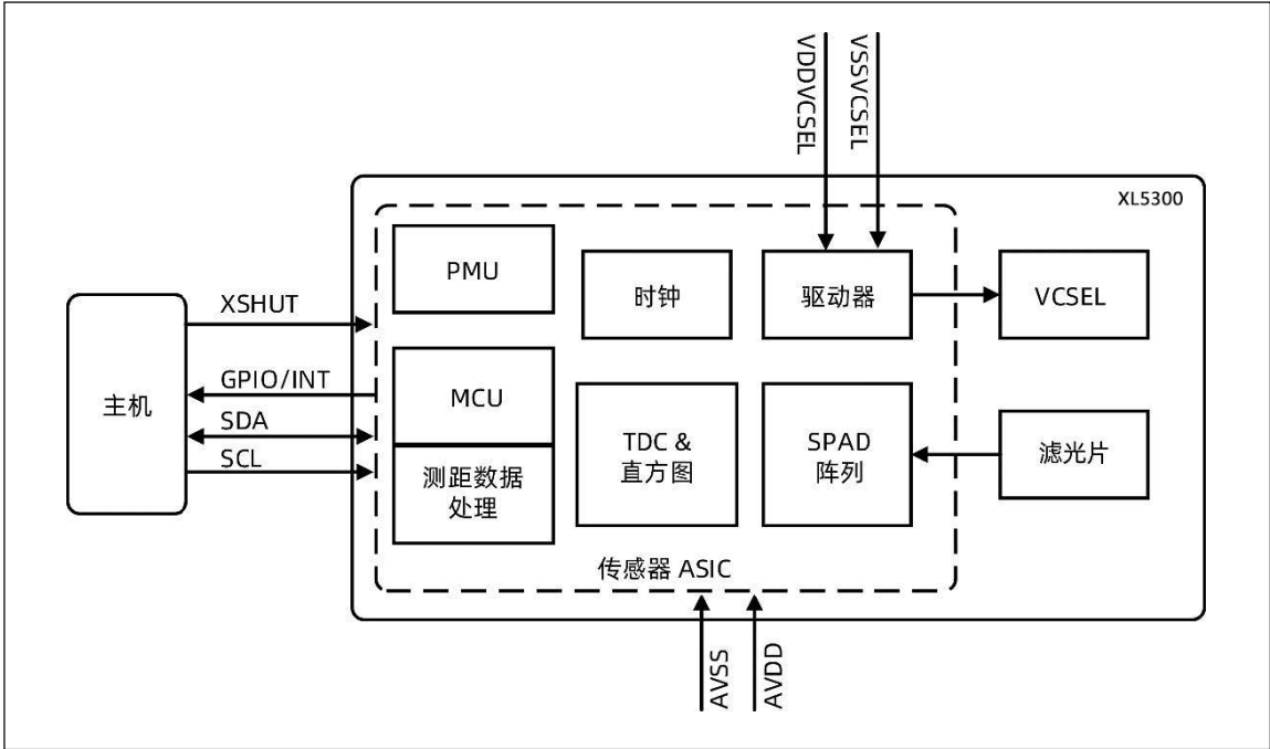
图 1：系统框图
