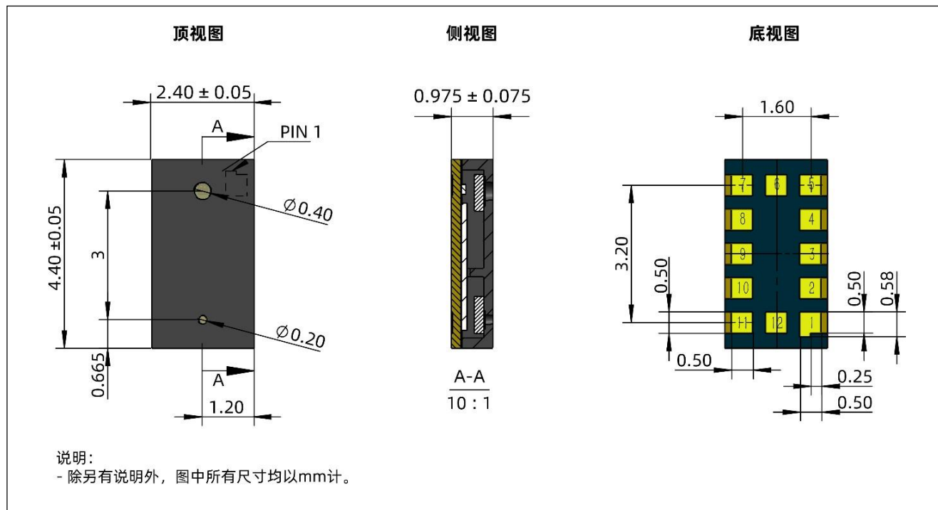
图 3 : XL5300 外形尺寸
