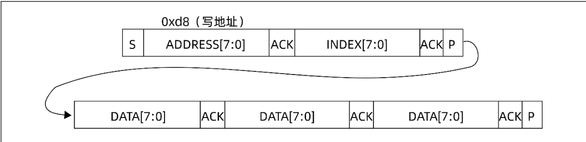
图 8 : XL5300 连续写数据格式
