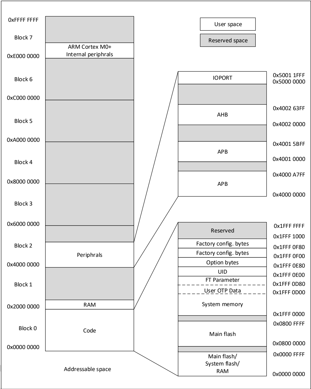
图 4-1 存储器映射
