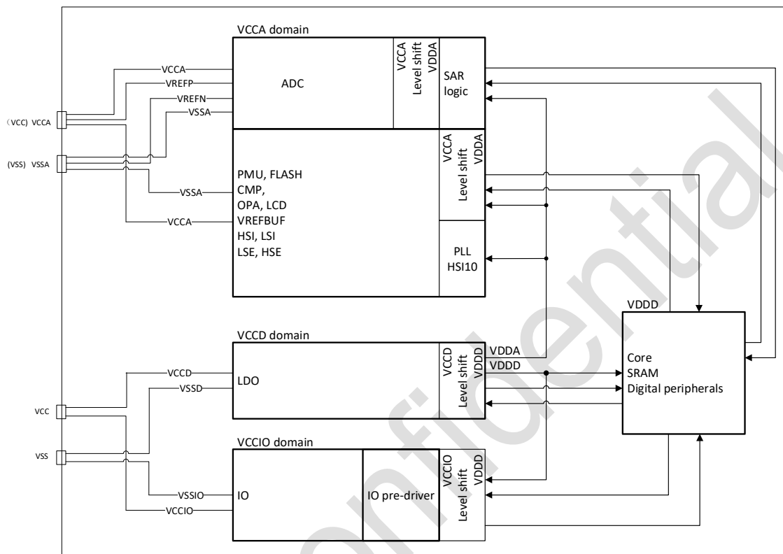
图 2-2 电源框图
