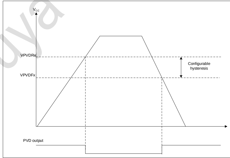
图 2-4 PVD 阈值
