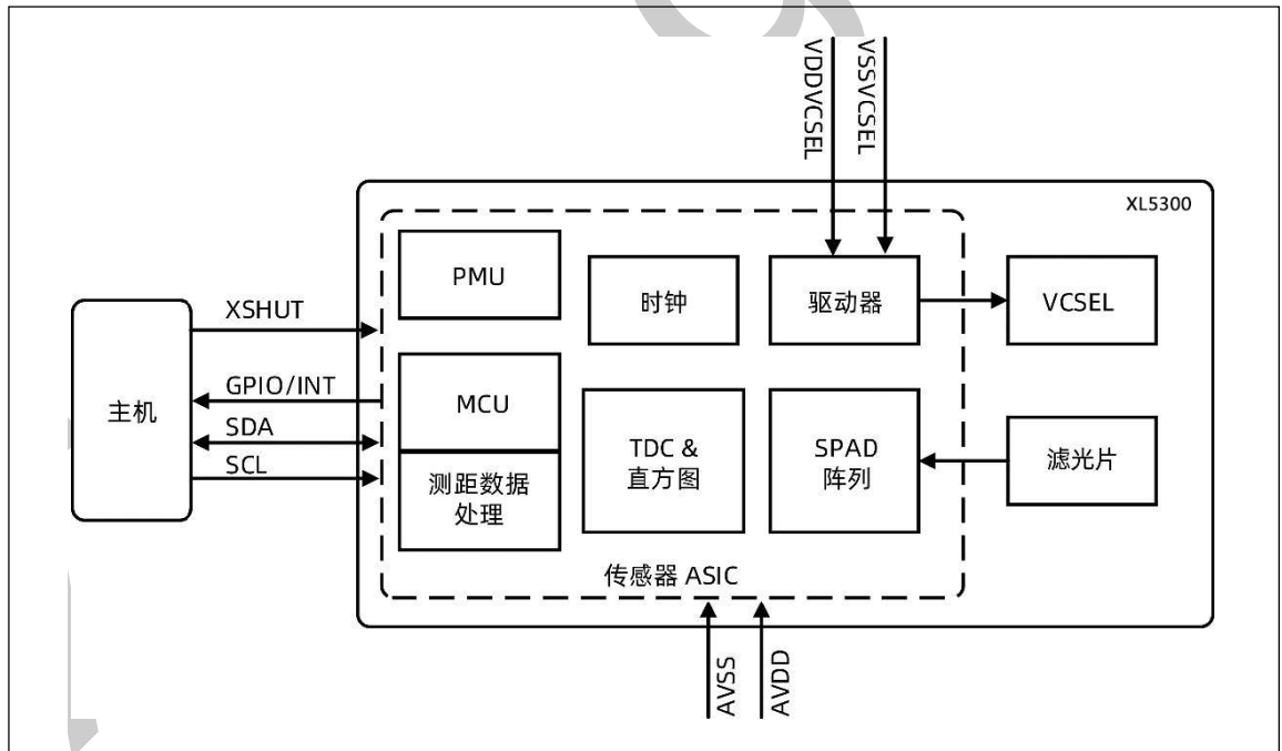
图 1：系统框图
