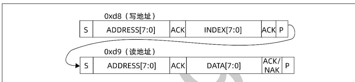
图 7 : XL5300 读数据格式
