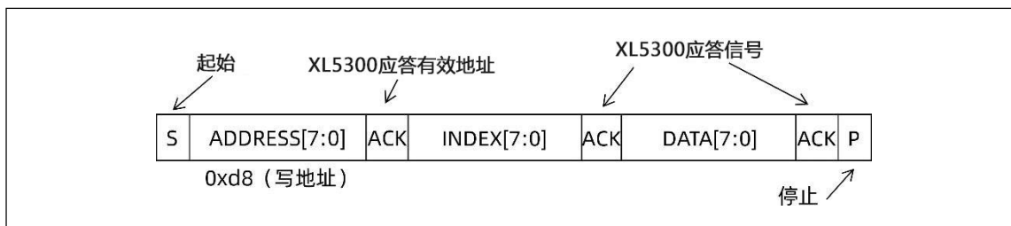
图 6 : XL5300 写数据格式
