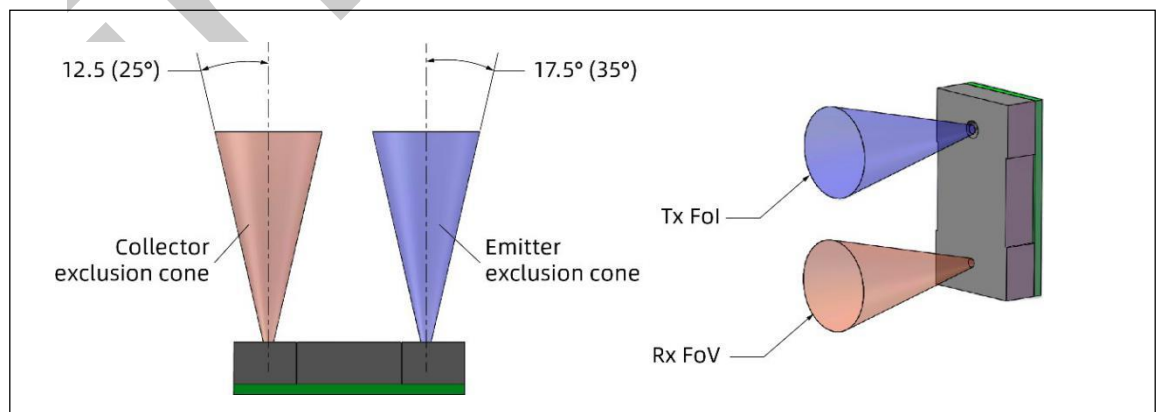
图 12 : XL5300 FoI/FoV
