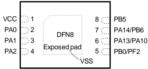
图 4-1 DFN8 PY32F003L2XD
