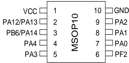
图 3-1 MSOP10 PY32F003A18N
