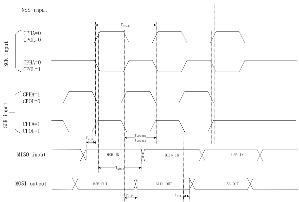
图 5-3 SPI 时序图—master mode
