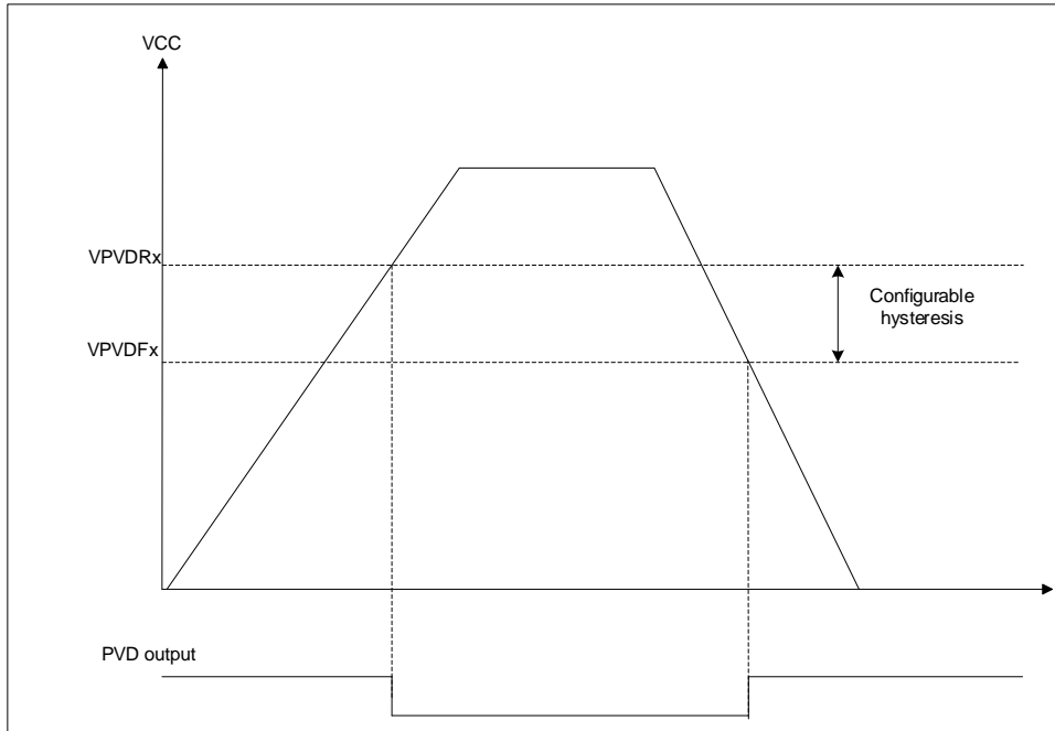
图 2-4 PVD 阈值
