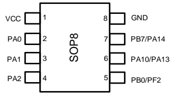
图 3-1 SOP8 PY32F003L2xS
