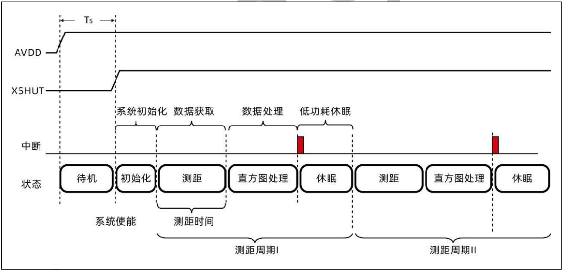
测距时序图
