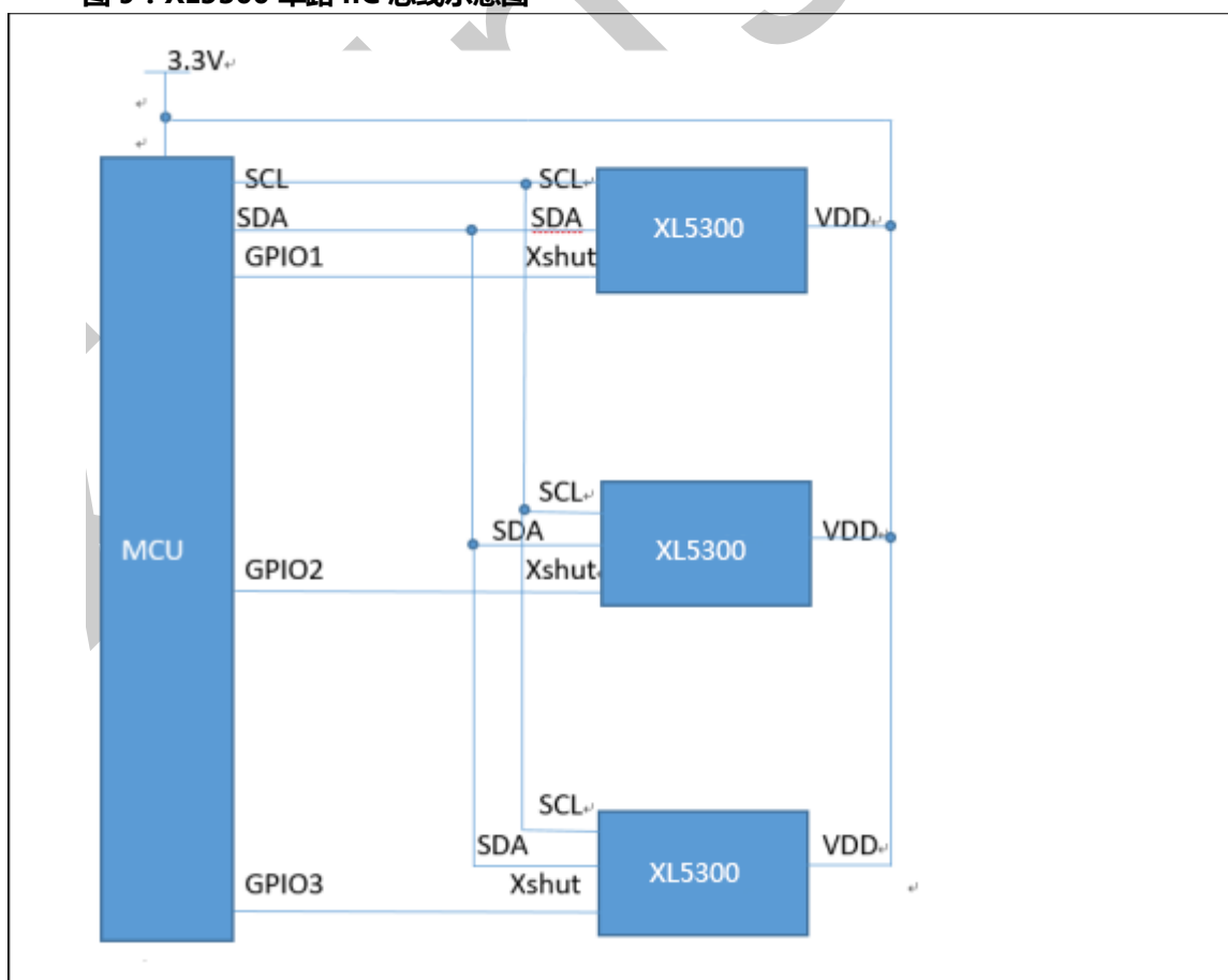
图 9：XL5300 单路 IIC 总线示意图
