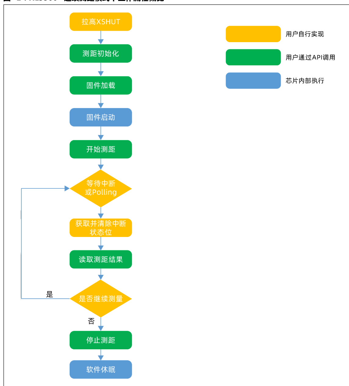
图 2：XL5300 连续测距模式下工作流程概览
