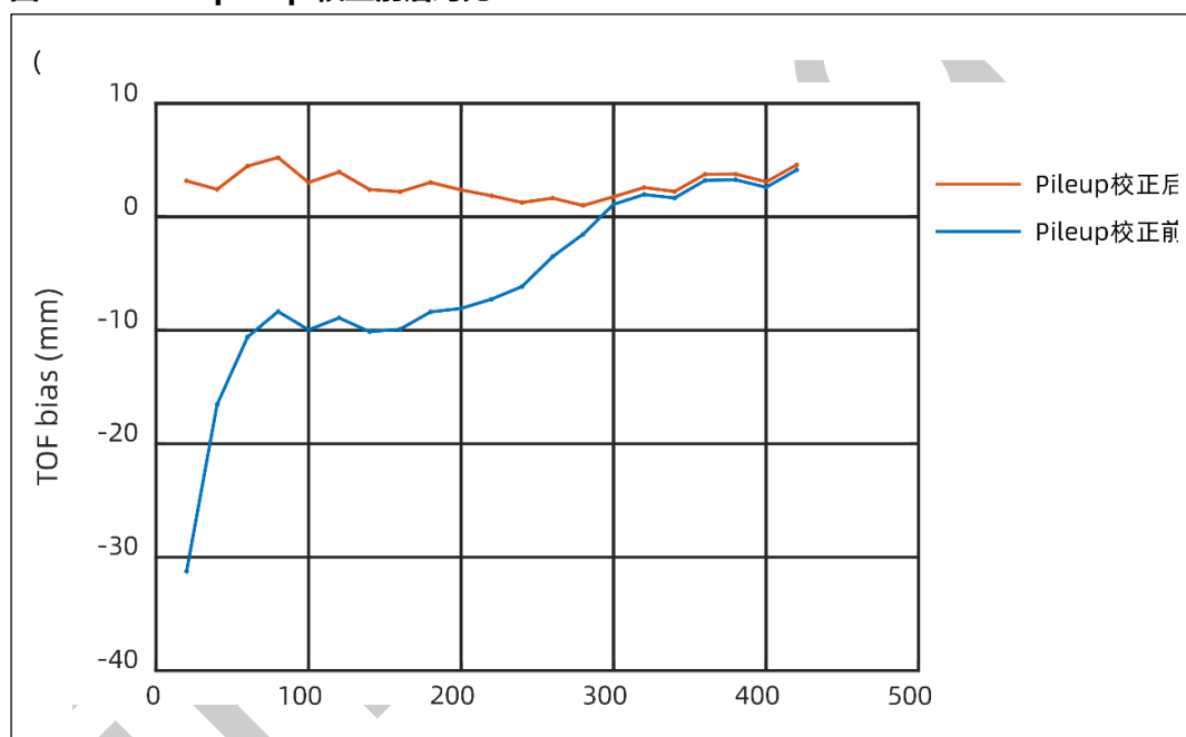
图 7：XL5300 pileup 校正前后对比
