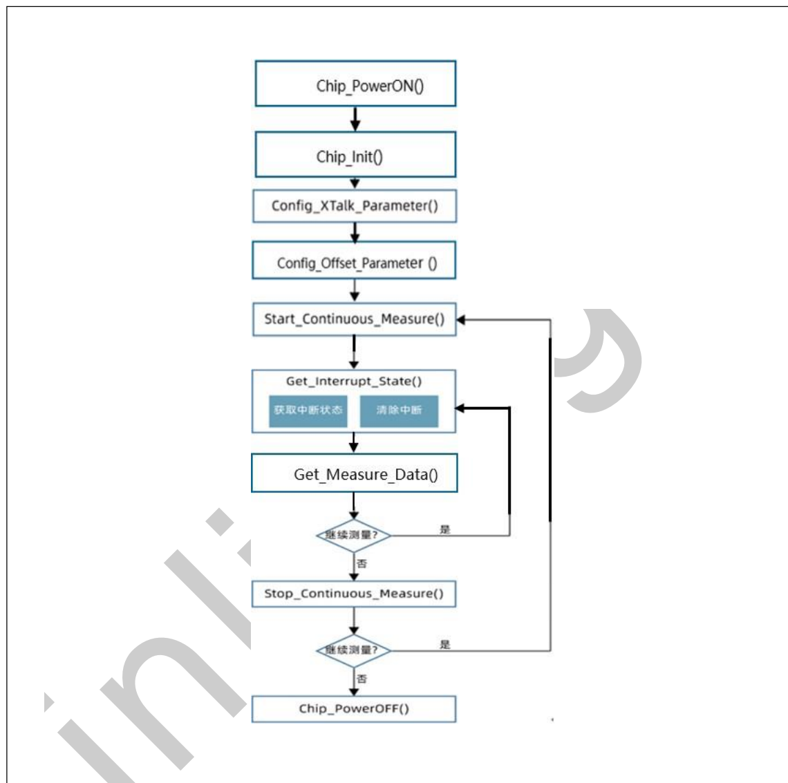
图 5：XL5300 API 测距流程
