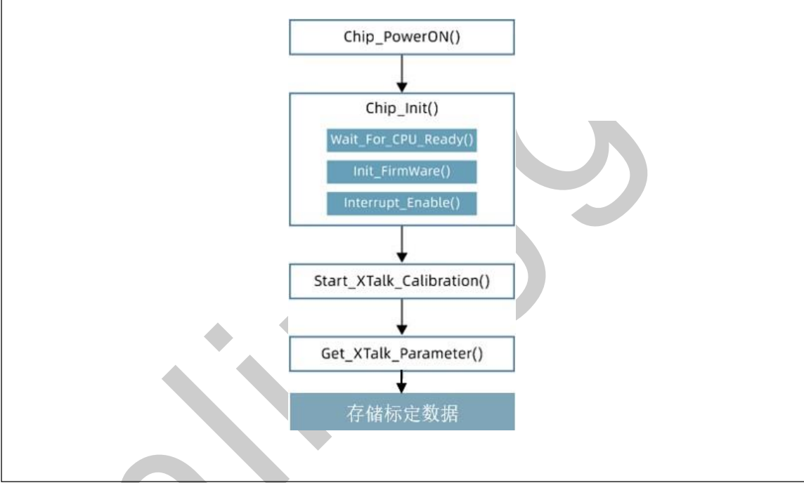
图 4：XL5300 API Offset 标定流程
