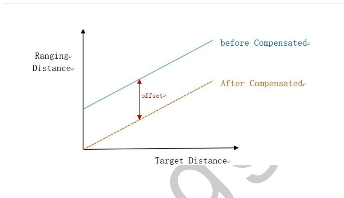
图 6 : XL5300 offset 标定对比图
