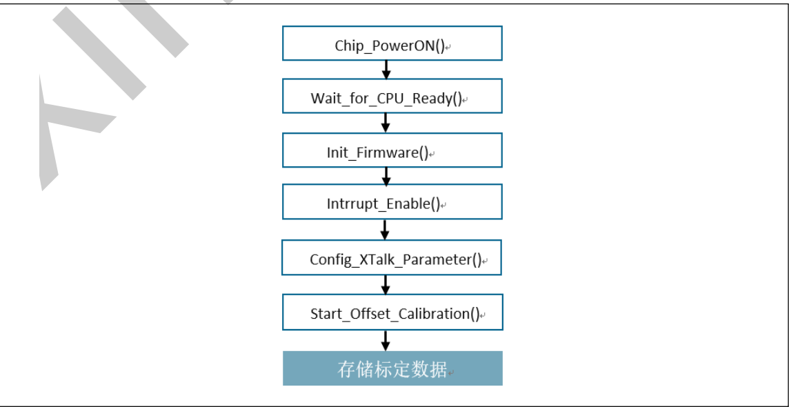
图 4：XL5300 API Offset 标定流程
