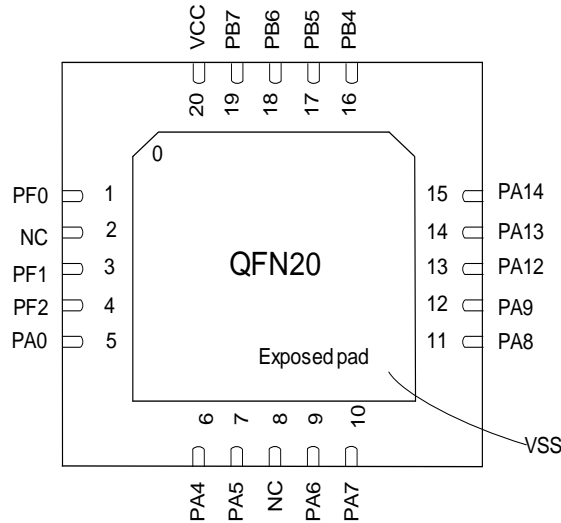
图 4-1 QFN20 Pinout3 PY32F030F3xU
